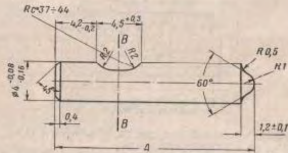
Рис. 36. Боек (удлиненный)
