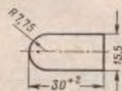
Рис. 81. Разделка паза для вклейки
