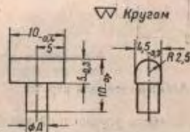
Рис. 16. Упор пружины колпачка
