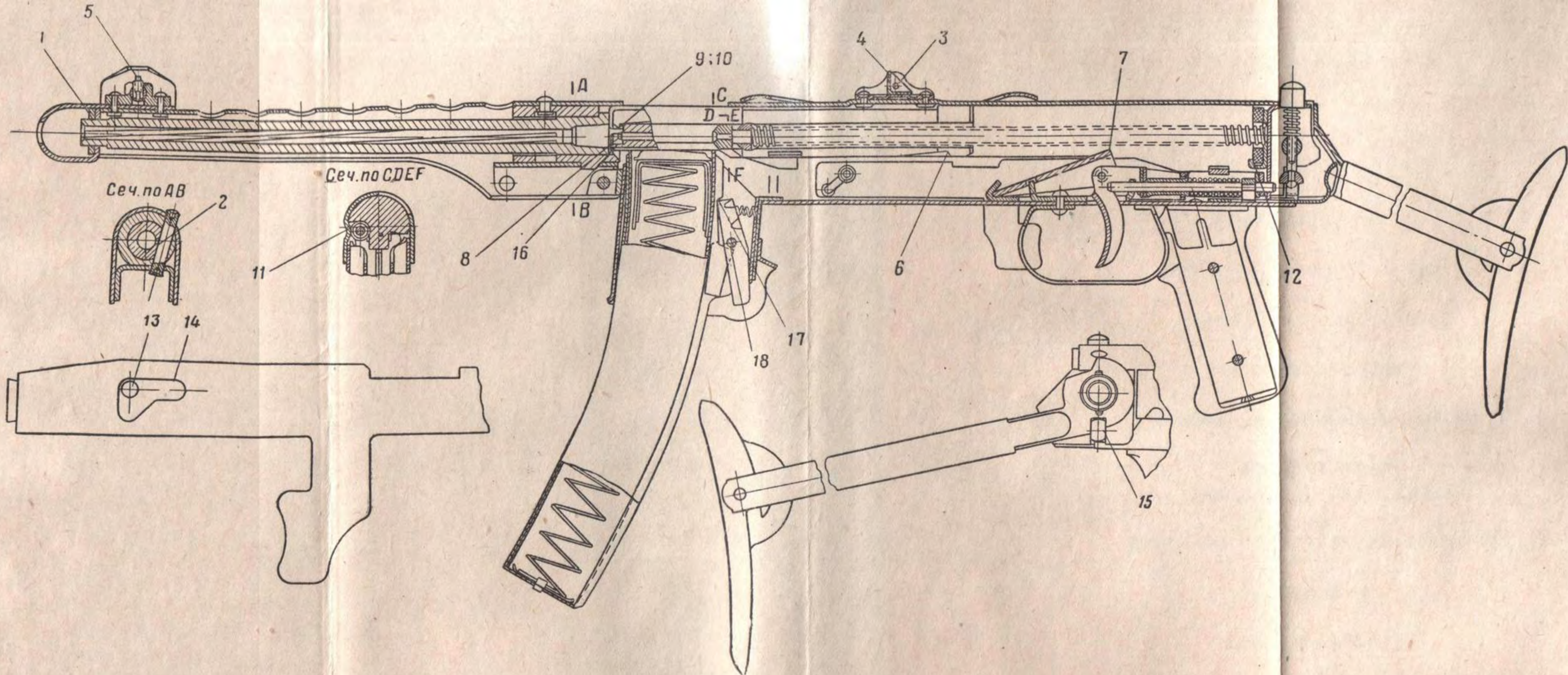
Черт. 2. 7,62-мм автомат (пистолет-пулемет) обр. 1943 г.
