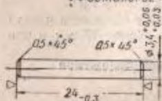
Рис. 24. Ось целика
