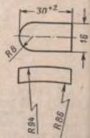
Рис. 78. Заготовка вклейки
