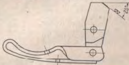
Рис. 32. Восстановление рабочей грани защелки магазина
