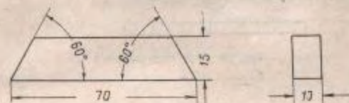
Рис. 54. Заготовка вклейки
