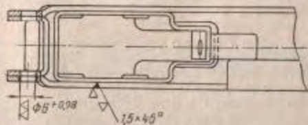
Рис. 135. Приварка вставки и спусковой коробки
