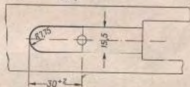
Рис. 81. Разделка паза для вклейки
