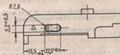
Рис. 21. Распиловка выреза в ствольной коробке под штифт защелки
