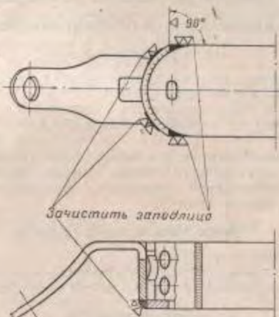
Рис. 31. Приварка хвостовика к затворной коробке
