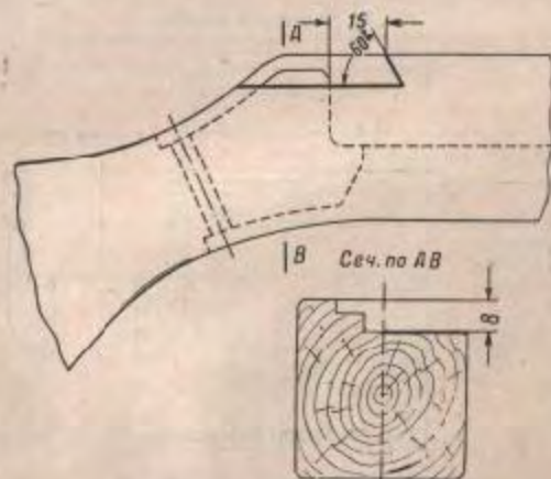
Рис. 57. Разделка паза для вклейки
