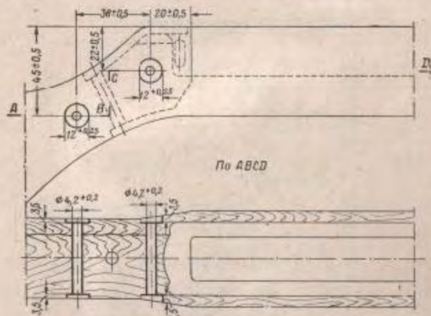
Рис. 73. Подготовка ложки для постановки нагелей
