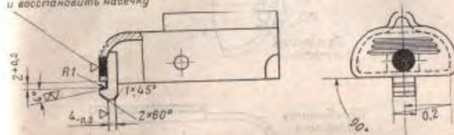
Рис. 20. Приварка зацепа к колпачку
