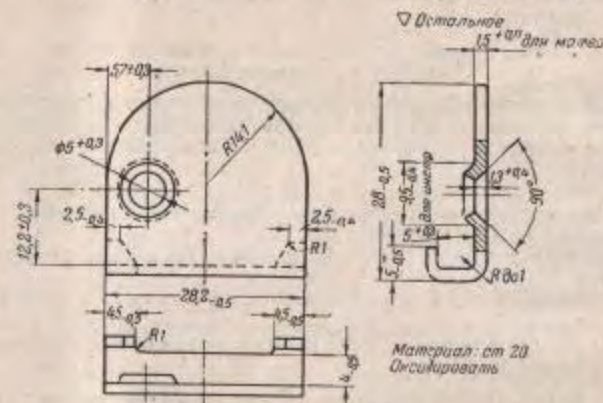
Рис. 142. Обойма амортизатора
