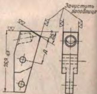
Острые ребра притупить R=0.3 Оксидировать
