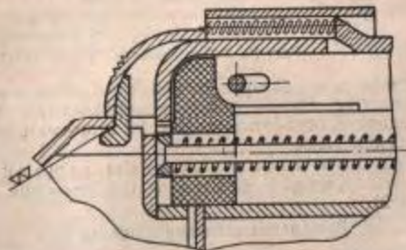
Рис. 17. Припиловка плоскости зуба зацепа
