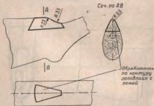
Рис. 91. Обработка вклейки
