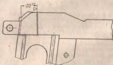
Рис. 134. Вставка
