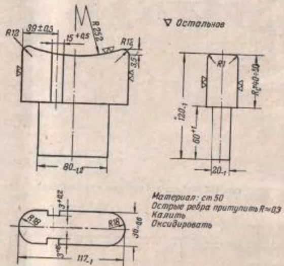
Рис. 175. Оправка для правки плечевого упора
