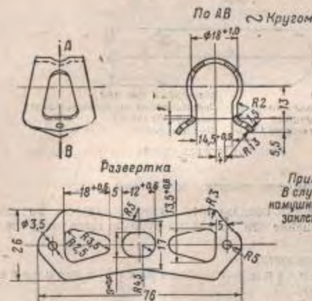
Рис. 25. Намушник
