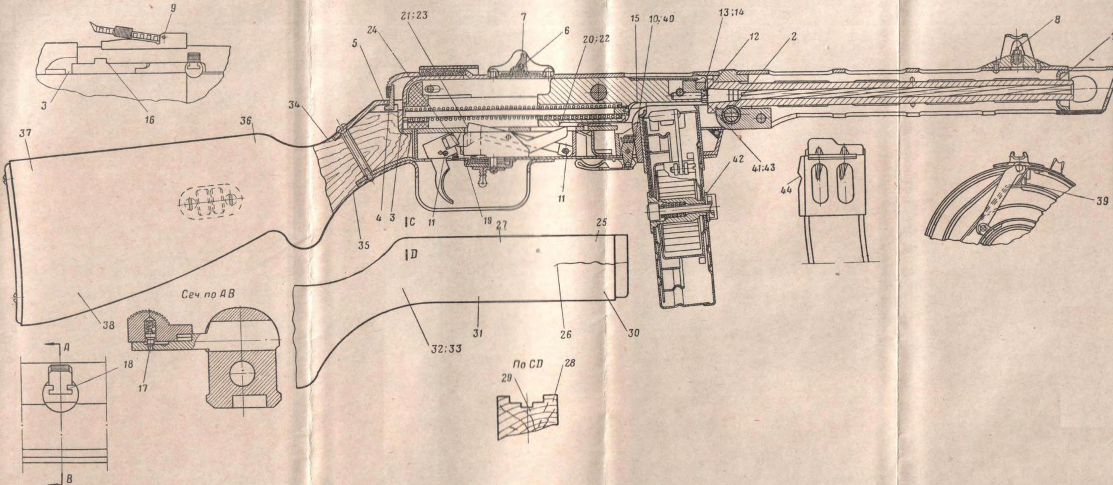
Черт. 1. 7,62-мм автомат (пистолет-пулемет) обр. 1941 г.
