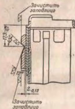
Рис. 115. Обработка выступа магазина
