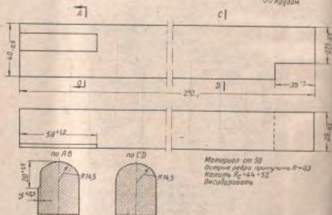
Рис. 172. Оправка для правки ствольной коробки
