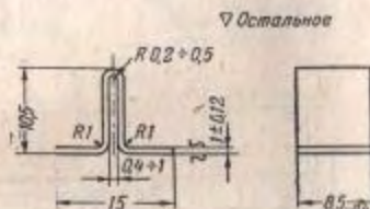
Рис. 111. Ограничительный выступ (пластичный)
