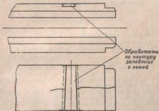
Рис. 52. Обработка вклейки
