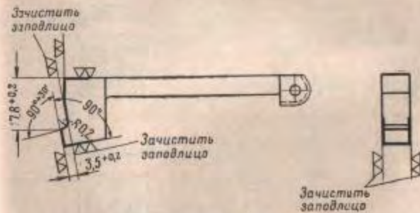
Рис. 40. Обработка спускового рычага
