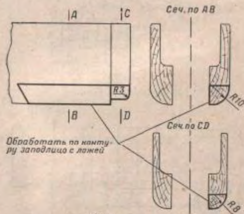
Рис. 68. Обработка вклейки
