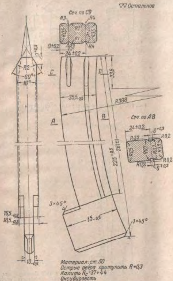
Рис. 165. Оправка для правки коромыслового механизма
