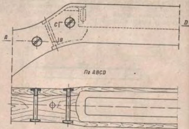
Рис. 76. Скрепление ложи нагелями
