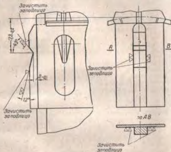
Рис. 117. Обработка выступа магазина
