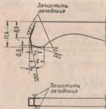
Рис. 43. Обработка разобщителя
