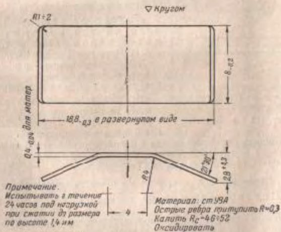
Рис. 131. Пруссина целика
