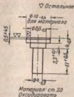
Рис. 148. Ось плечевого упора
