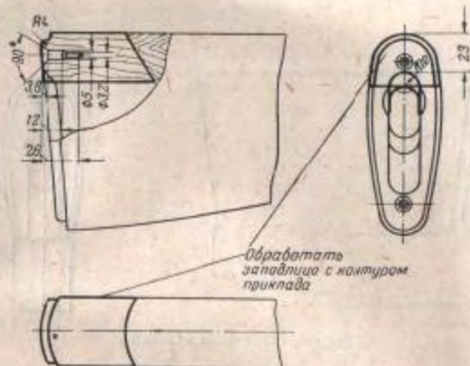
Рис. 95. Обработка вклейки
