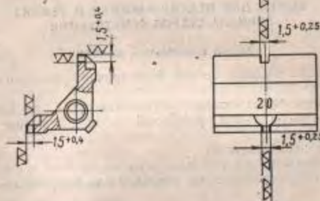
Рис. 28. Опиловка гнилок и прорезей целика
