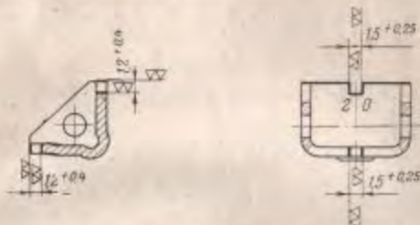
Рис. 133. Опилки гривок и прорезей целика
