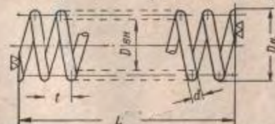
Материал: проволока „В“ ГОСТ 5047-49
