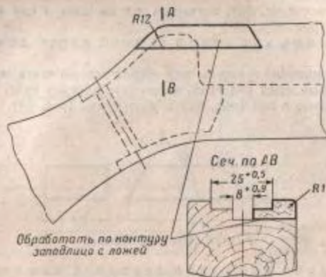
Рис. 60. Обработка вклейки
