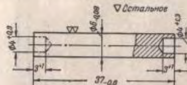
Рис. 126. Запарка отвёрстия вкладыша под заклепку
