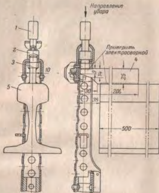
Рис. 123. Подсадка отверстия в передней стенке направляющей ствола
