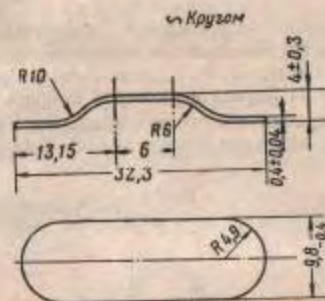
Рис. 23. Пружина целика
