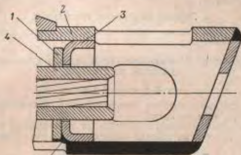
Рис. 9. Приварка направляющей планки к передней направляющей ствола:
