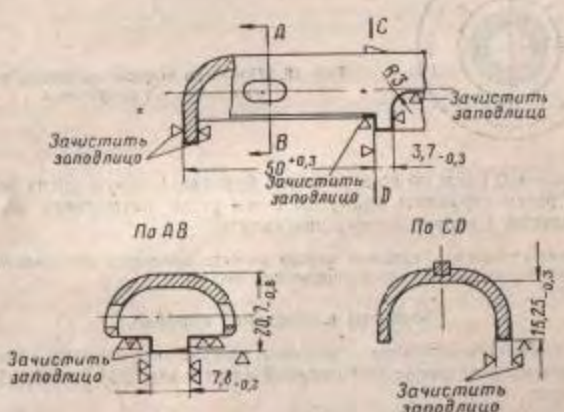
Рис. 12. Обработка выступа и правого уступа ствольной коробки
