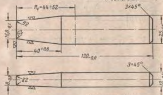
Материал: ст. 50 Острые ребра притупить R \approx 0,3 Калить Окисливать
