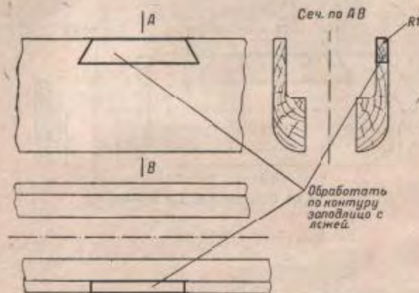
Рис. 56. Обработка вклейки
