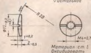
Рис. 75. Гайка нагеля
