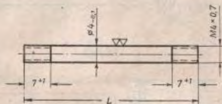
Рис. 74. Стержень нагеля
