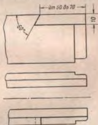
Рис. 45. Разделка паза для вклейки
