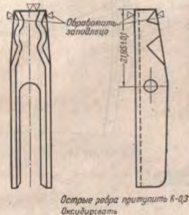
Рис. 152. Обработка защелки магазина
