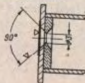
Рис. 109. Приклепка ограничительного выступа к улитке
