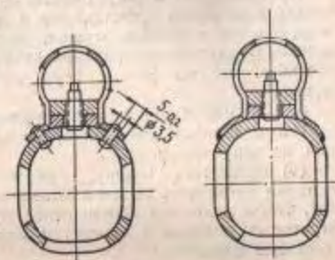
Рис. 27. Приварка намушника
