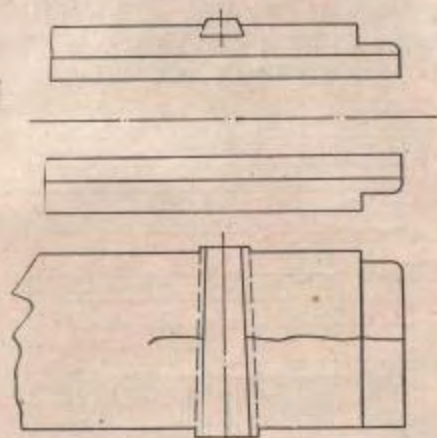
Рис. 51. Постановка вклейки
