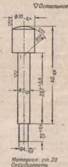
Рис. 149. Кнопка
