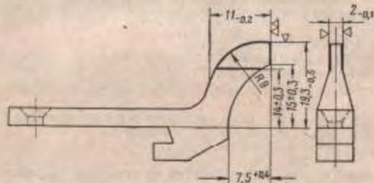
Рис. 38. Сработка верхней части отражателя старой конструкции
