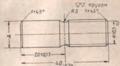
Рис. 2. Упрощенная ось ствольной коробки
