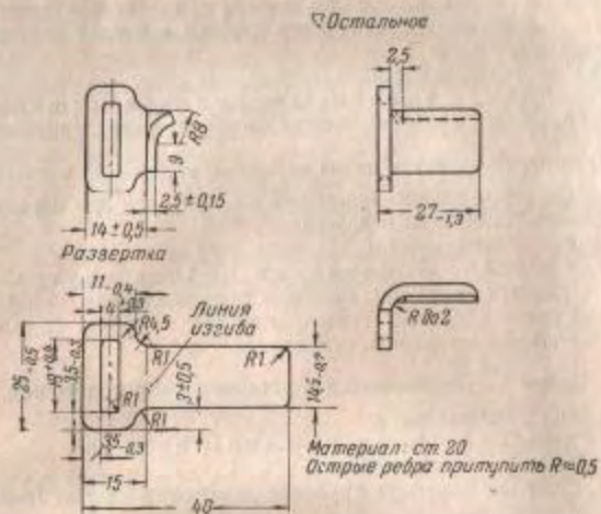
Рис. 130. Антубка ствольной коробки
