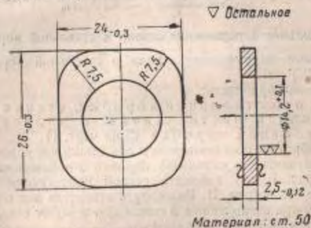
Рис. 8. Направляющая планка
