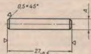
Рис. 44. Штифт бойка
