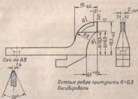
Рис. 37. Обработка верхней части отражателя
