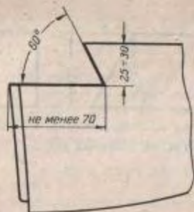
Рис. 92. Разделка паза для вклейки
