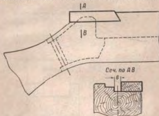
Рис. 59. Постановка вклейки
