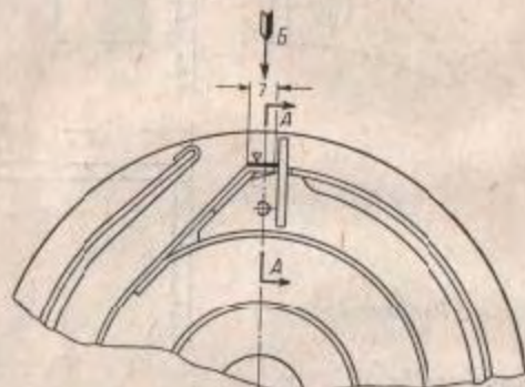
Рис. 108. Заклепка
