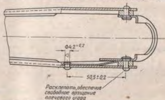
Рис. 147. Приклепка пружины и замена осей плечевого упора
