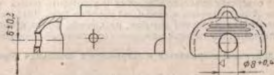
Рис. 18. Подготовка колпачка для приварки зацепа
