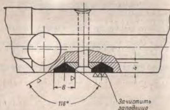
Рис. 143. Приварка рукоятки затвора
