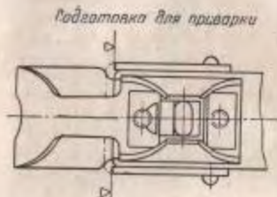
Рис. 125. Приварка направляющей планки к направляющей ствола
