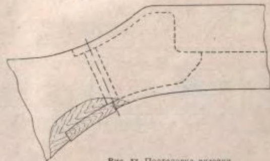
Рис. 83. Поставовка вклейки
