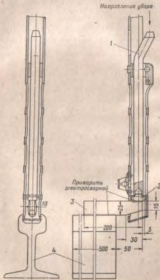
Рис. 7. Подсадка отверстия в передней направляющей: 1 — гильза; 2 — подставка; 3 — болос; 4 — рельс
