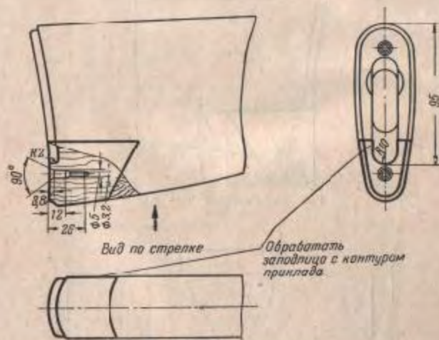
Рис. 99. Обработка вклейки
