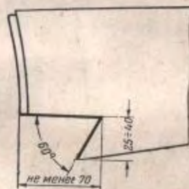
Рис. 96. Разделка паза для вклейки
