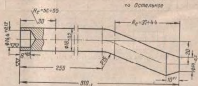
Рис. 164. Гнезко для посадки отверстия в передней направляющей ствола
