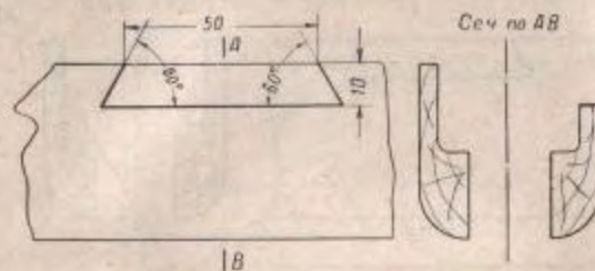
Рис. 53. Разделка паза для вклейки
