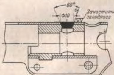
Рис. 126. Запарка отвёрстия вкладыша под заклепку
