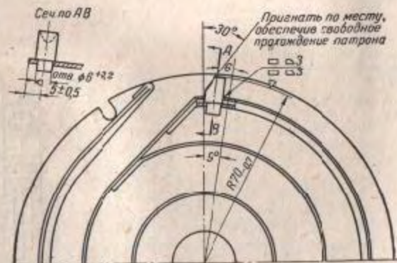
Рис. 112. Приварка ограничительного выступа (цилиндрического)
