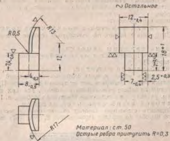
Рис. 19. Зацеп защелки
